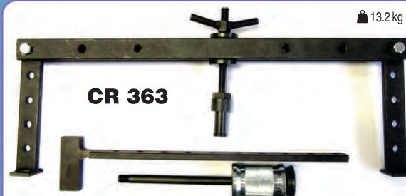
Dispositivos para retirar bico injetor eletrônico. Carretel Rosca M27 X 1mm. Sistema (sacador com rosca) em linha, ou individual no sistema (à percussão) Acompanha adaptador para Renault Master (apoiar na caixa seca do câmbio). OBS: Os bicos devem ser de rosca M27 X 1mm e estar sem o solenóide, em condições normais.
